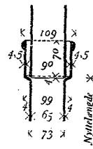
Muffedimensioner for 65 mm (2 1/2") Faldrør.
