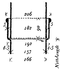
Muffedimensioner for 157 mm (6") Faldrør.
