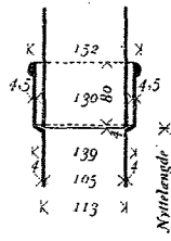
Muffedimensioner for 105 mm (4") Faldrør.
